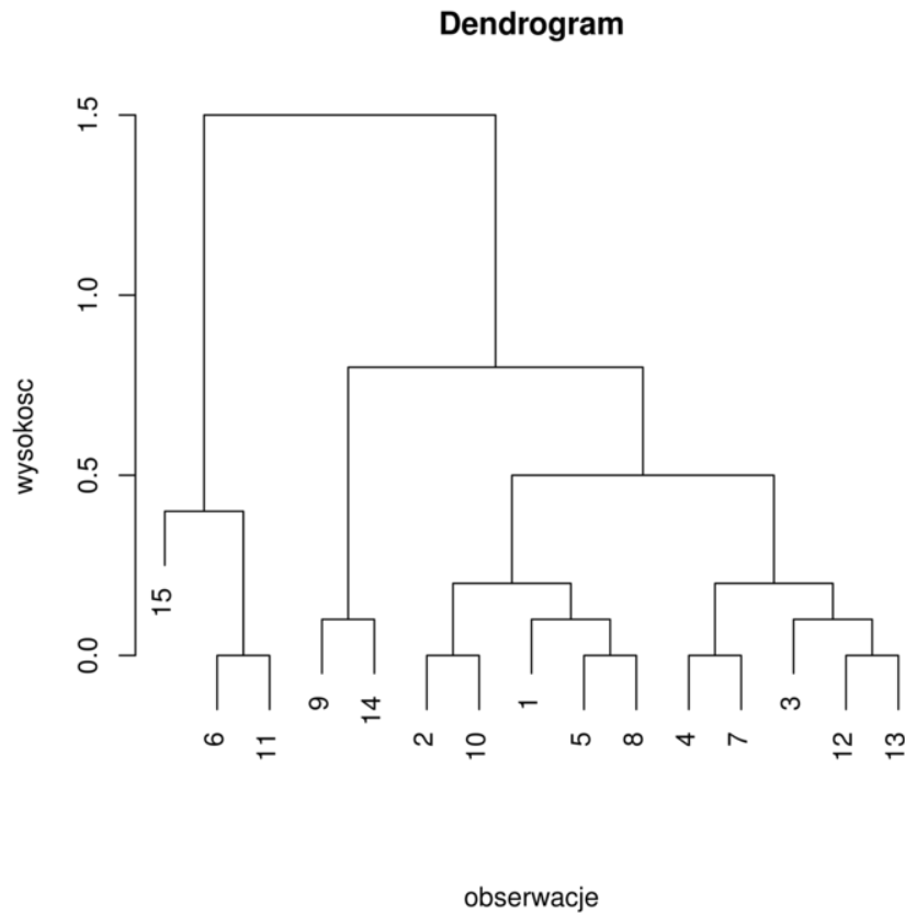
Rysunek 6.2. Przykładowy dendrogram dla klasteryzacji hierarchicznej.
