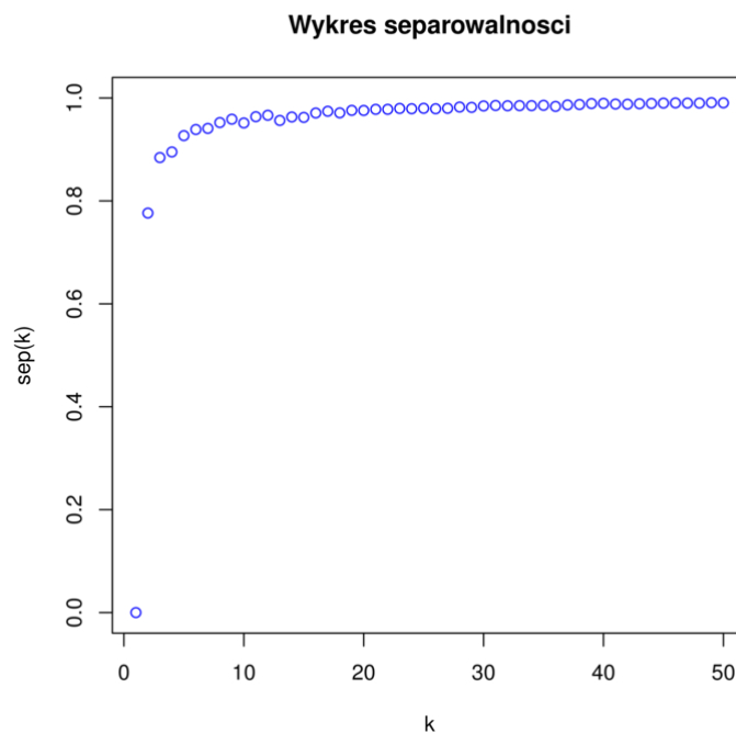
Rysunek 6.3. Przykładowy wykres separowalności dla danych Iris.
