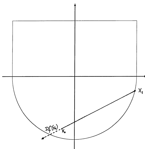
Rysunek 14.3. Ilustracja problemu ze znalezieniem kierunku dopuszczalnego największego spadku.
